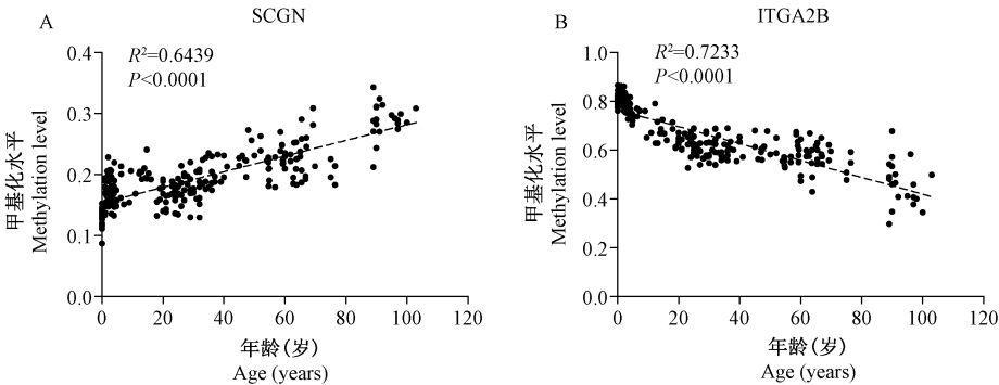
注:A:SCGN 甲基化水平与年龄呈正相关;B:ITGA2B 甲基化水平与年龄呈负相关。
