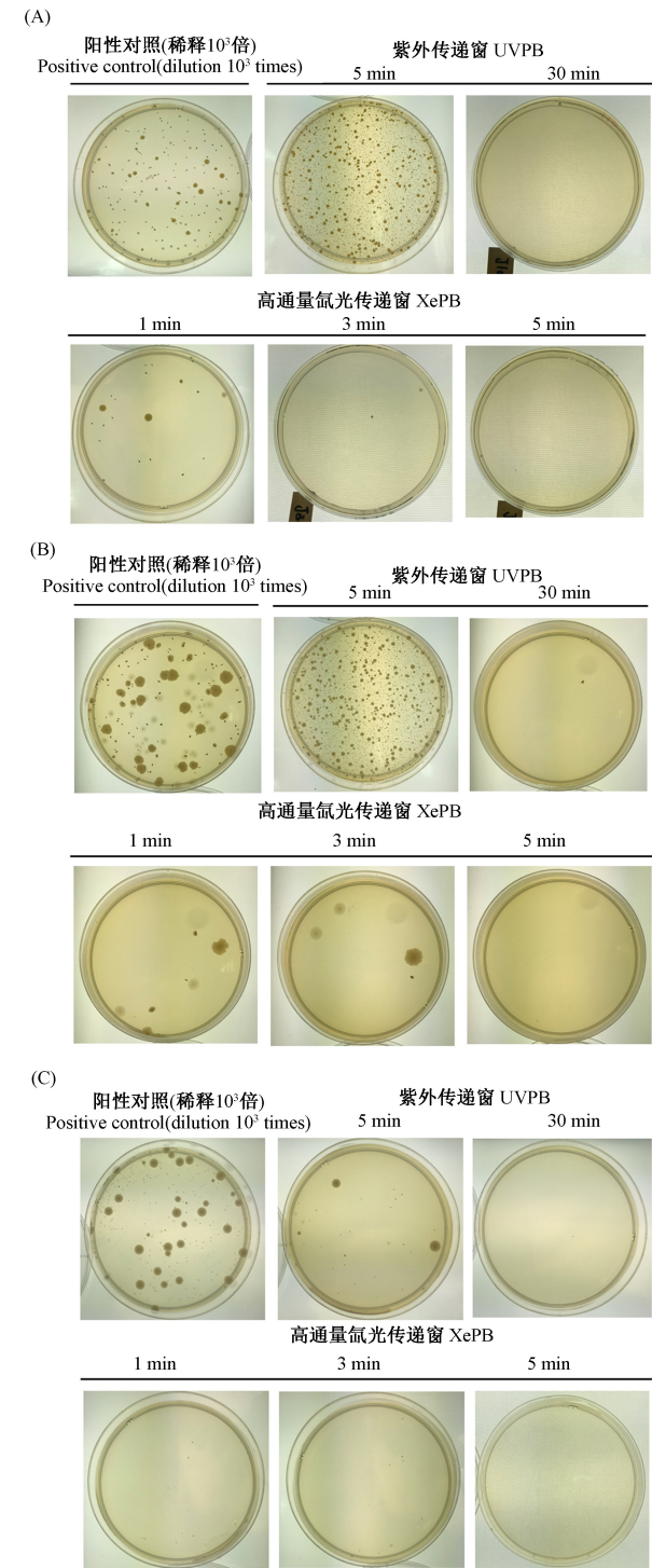
注: A;金黄色葡萄球菌;B:大肠杆菌;C:绿脓杆菌;阳性对照:阳性洗脱液稀释后铺板,培养 48 h。 图 1 紫外传递窗和高通量氙光传递窗在不同照射时间点对金葡、大肠、绿脓的悬液涂布照射结果 Note. A, Staphylococcus aureus . B, Escherichia coli . C, Pseudomonas aeruginosa . Positive control, The positive eluent was cultured 48 h after dilution.
