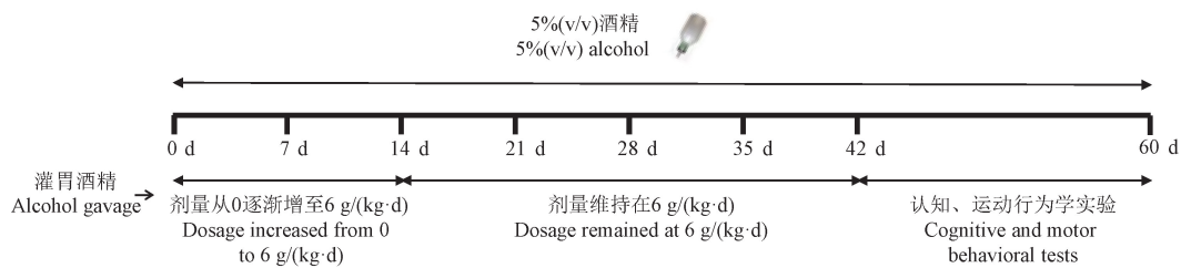
图 1 慢性酒精中毒性脑损伤的建模过程和行为学实验时间表
