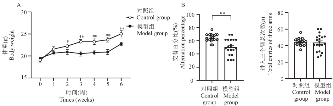
图2 小鼠体重和 Y 迷宫实验结果比较
