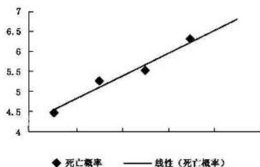
图 C.1 浓度对数和死亡概率单位关系图
