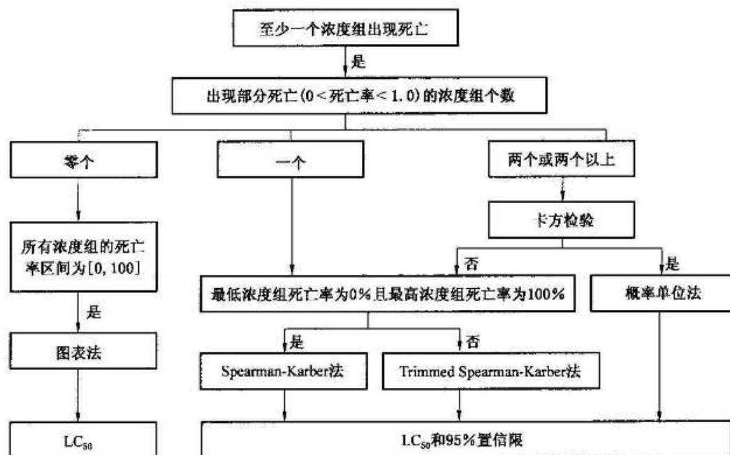
图 B.2 LC_{50} 的计算流程
